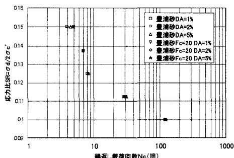
図 3 応力比～繰返し載荷回数の関係 ( Dr=40\% )
