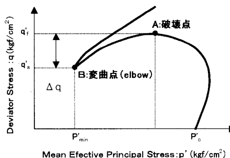
Fig. 2 応力経路
