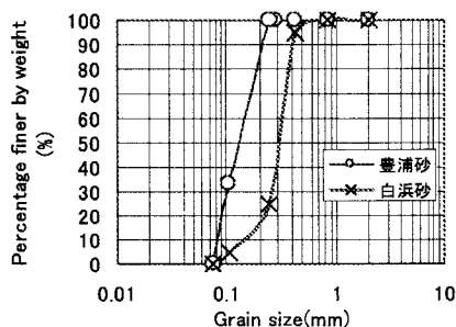
Fig. 1 粒径加積曲線
