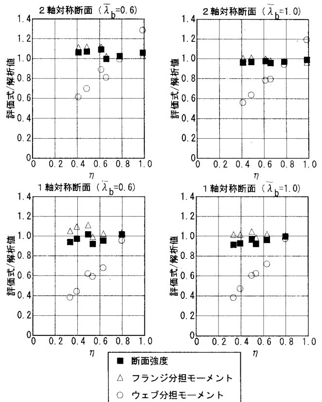
図-3 減衰係数 \eta による強度評価式の評価
