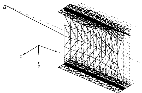
図-1 初期たわみ図
