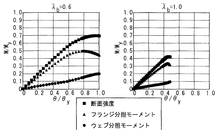
図-2 モーメントと強制回転角の関係
