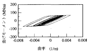
(b) 水平反力分散支承
