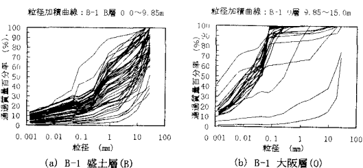
図 2 粒径加積曲線の一例
