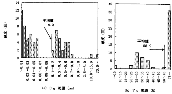
図 3(b) O 層における D_{50} , F_c の頻度
