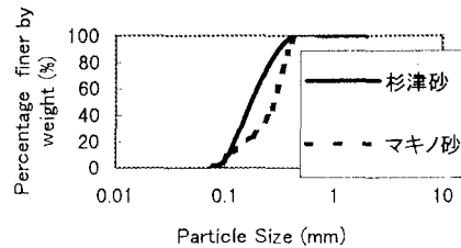
Fig.1 粒径加積曲線
