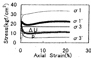
Fig.4(c) 応力-ひずみ関係 ( R_c < 2 )
