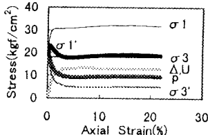
Fig.4(b) 応力-ひずみ関係 ( R_c = 2 )
