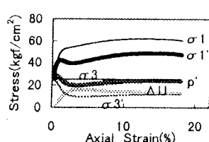
Fig.3(c) 応力-ひずみ関係 ( R_c < 2 )
