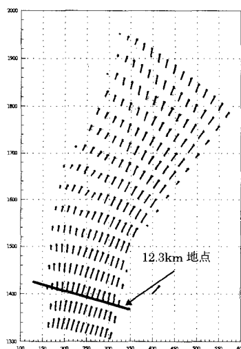
図8 10時間後の 流速ベクトル（植生なし）
