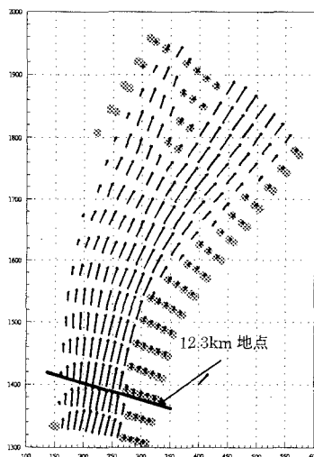
図7 10時間後の 流速ベクトル（植生固定）
