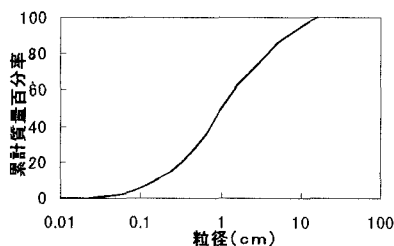
図4 粒度分布
