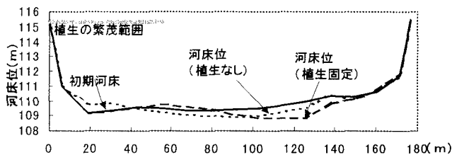
図5 64時間後の河床横断形状
