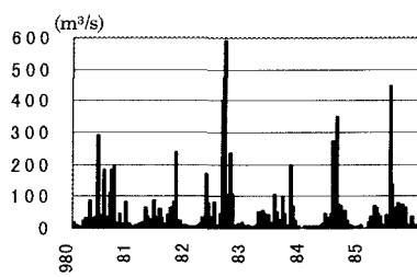
図2 1980~1985年の日平均流量
