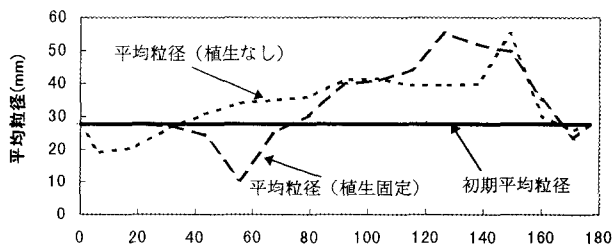
図6 64時間後の平均粒径の横断分布
