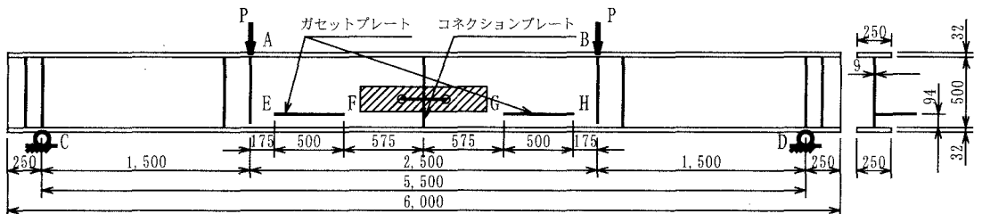
図-2 桁試験体詳細図
