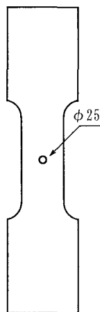
図-6 円孔を有する帯板試験片
