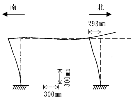
図-5 ピーク 6 のときの変形状況
