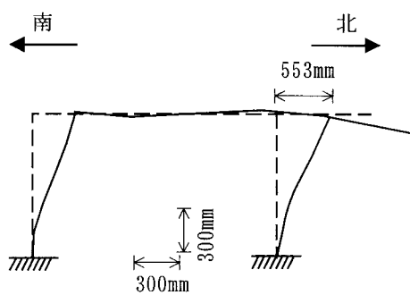
図-6 ピーク 9 のときの変形状況
