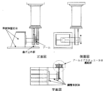
図-2 実験装置
