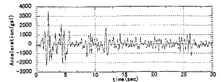
図 4 加振機に力する加速度
