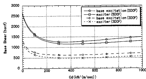
図 7 各フレームのベースシアの推移
