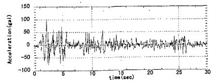
図 3 再現すべき地震動 (El Centro NS)
