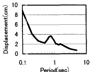
図7 橋脚が非線形のときの標識柱の最大変位応答スペクトル
