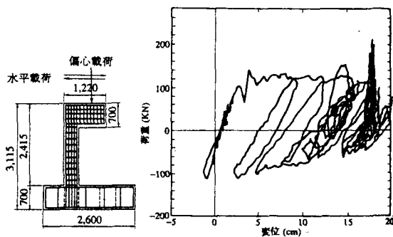
図-5 振動台実験から得られた荷重-変位の履歴[2]
