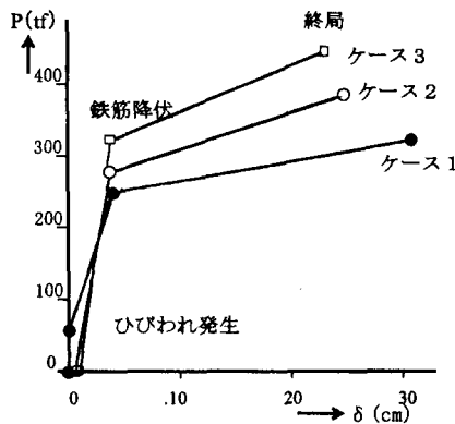
図-4 水平力(P)-上部工重心位置の水平変位(δ)の関係
