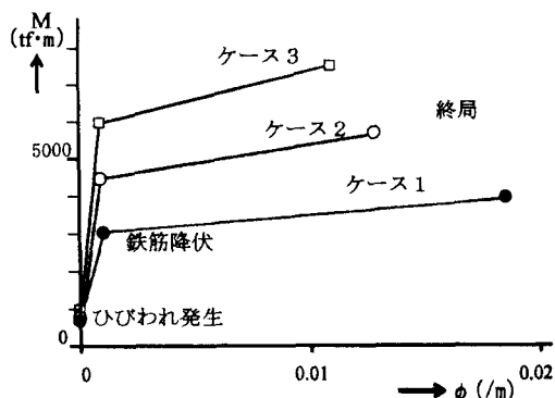
図-3 橋脚下端における曲げモーメント(M)-曲率(φ)の関係
