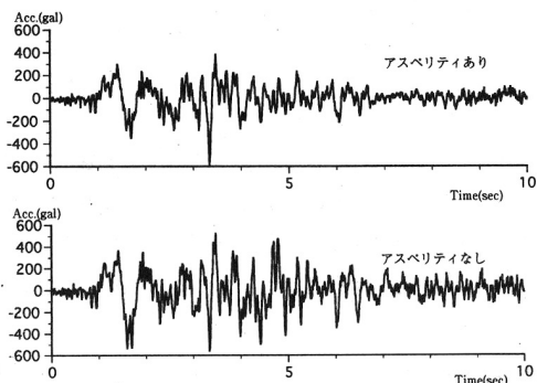
図2 アスベリティの有無による地震波の相違
