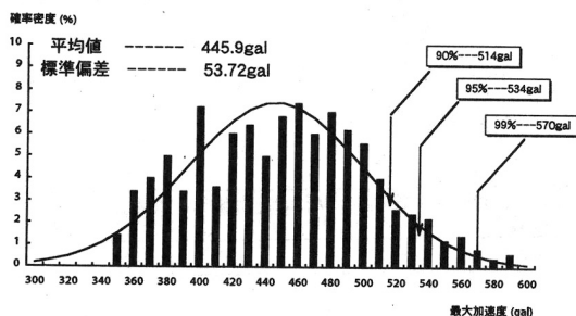
図3 アスベリティによる最大加速度のばらつき
