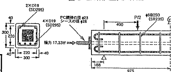
図-2 せん断小型供試体諸元
