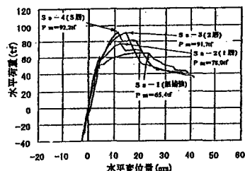
図-4 Sa シリーズ：荷重-変位曲線
