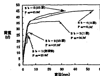
図-5 Sb シリーズ：荷重-変位曲線
