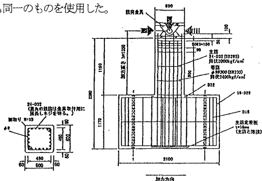
図-1 せん断大型供試体諸元
