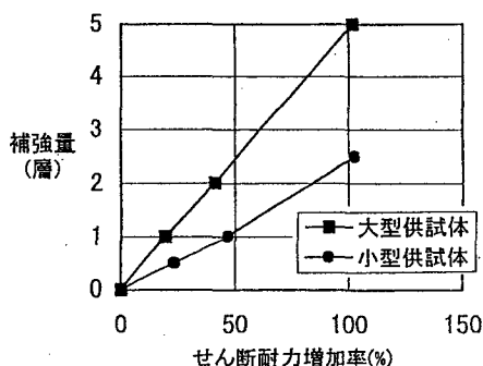
図-6 セン断耐力増加率比較図
