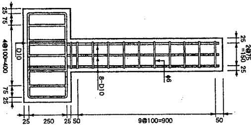
図 1 代表的な供試体形状
