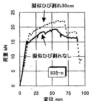
図 2-3 ひび割れと段落し
