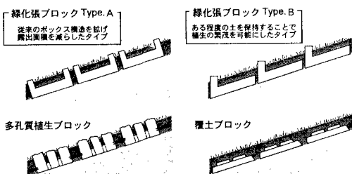
図-4 「植生」を意識したブロック
