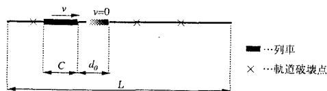
図1 理論解析モデル
