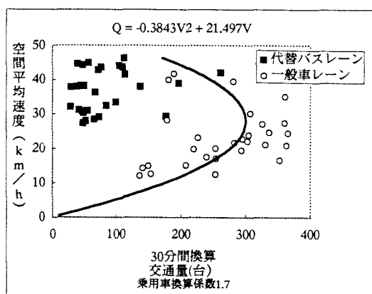
図-3 空間平均速度と交通量の相関図
