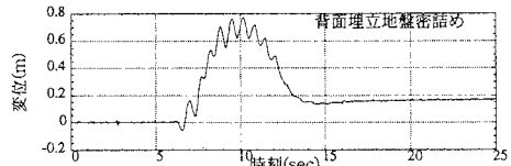
図-7 ケーソン水平変位
