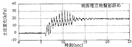
図-8 ケーソン下部土圧増分
