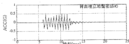
図-2 入力加速度
