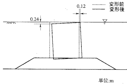
図-6 ケーソン最終変状 (背面埋立地盤密詰め)
