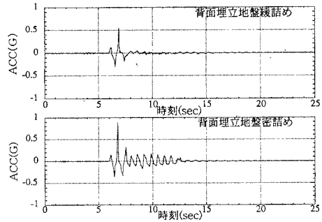
図-5 ケーソン水平方向加速度
