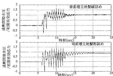
図-3 背面埋立地盤過剰間隙水圧比
