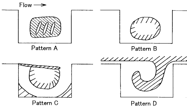
図-2 死水域内の浮遊砂堆積パターン
