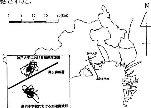
図-5 1997.01.08の地震記録(M=4.0 震源地：京都中部)
