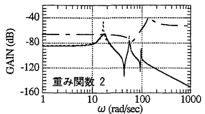
—— H_\infty 制御理論による伝達関数 --- 重み関数 ..... 無制御状態の伝達関数
