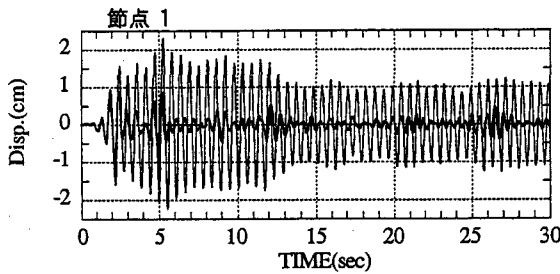
図4 H_{\infty} 制御による変位応答（制御遅れ0.04秒）
