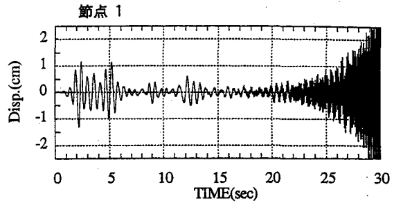
図3 LQ制御における変位応答（制御遅れ0.02秒）
