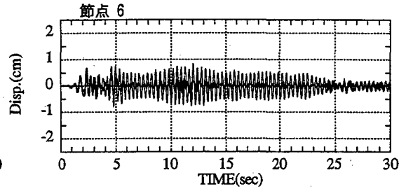
細線:無制御時 太線:制御時
