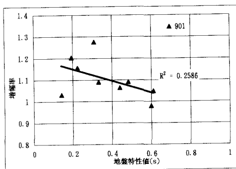
図-4.1 地盤卓越周期と増幅率
