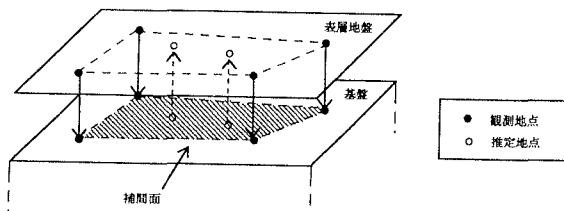
図-2.1 空間的広がり考慮した加速度推定
