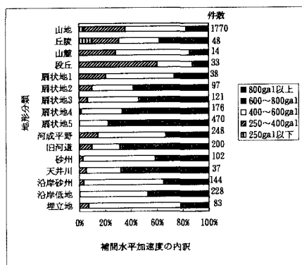
図-3.2 補間水平加速度と地形分類
