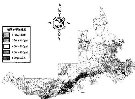
図-3.1 補間水平最大加速度分布
