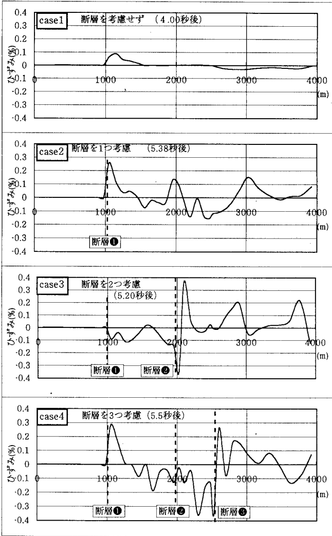
図4 最大ひずみ発生時刻での管頂ひずみ分布図
