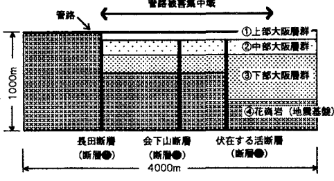
図1 解析モデル 表1 推定地質パラメータ
