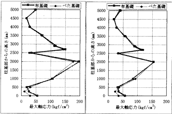
(a) 本山周辺地盤 (b) ポートアイランド 図3 通し柱最大軸応力 (地盤種別別)
