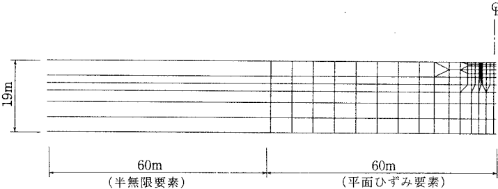
図1 地盤解析モデル
