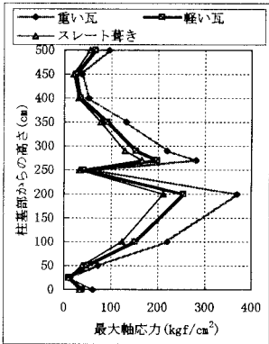
図4 通し柱最大軸応力 (屋根形式別)
