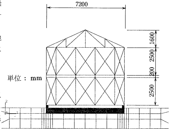
図2 建物、基礎および地盤モデル（拡大図）
