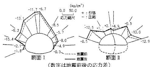
図6 吹付コンクリート応力分布の比較
