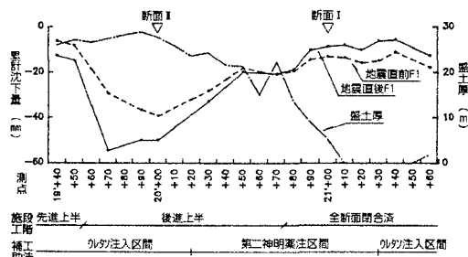
図5 地震前後の天端沈下量(F1)縦断分布
