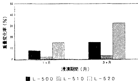
図1-L-500, 510, 520の浸漬後の重量変化率
