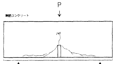
図-5 試験供試体
