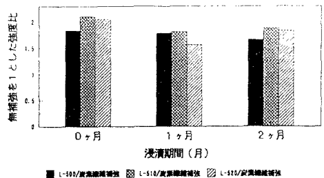
図8-CFRP補強コンクリートの曲げひび割れ発生荷重の浸漬による変化
