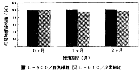
図4-CFRPの浸漬後の強度保持率
