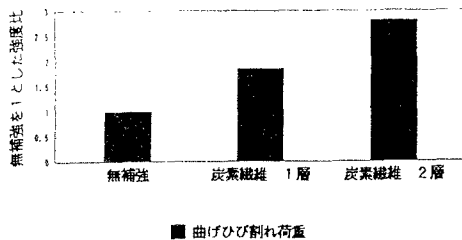
図7-炭素繊維補強による曲げひび割れ発生荷重
