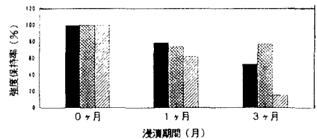
図2-L-500, 510, 520の浸漬後の引張強度保持率
