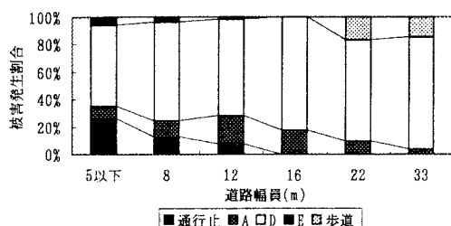
図-4 住吉地区道路幅員別被災状況
