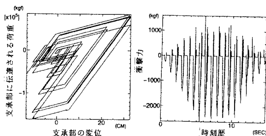
図-6 CASE2の支承部の変位-荷重履歴と 桁の衝突による衝撃力の時刻歴
