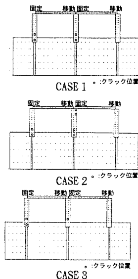
図-3 クラックの発生箇所
