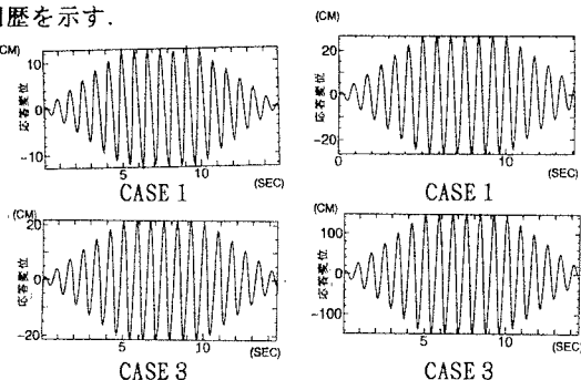
図-4 橋脚基部に対する図-5 基盤面に対する 天端部の応答変位 天端部の応答変位
