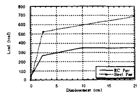
図-2 各橋脚の地震時保有水平耐力
