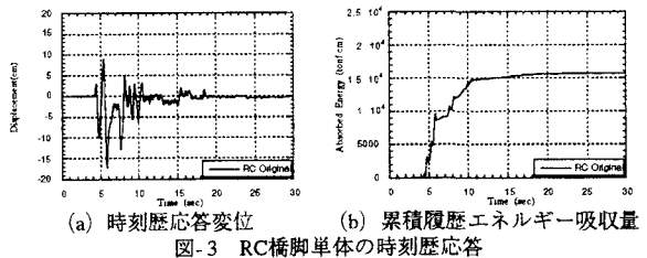
図-3 RC橋脚単体の時刻歴応答
