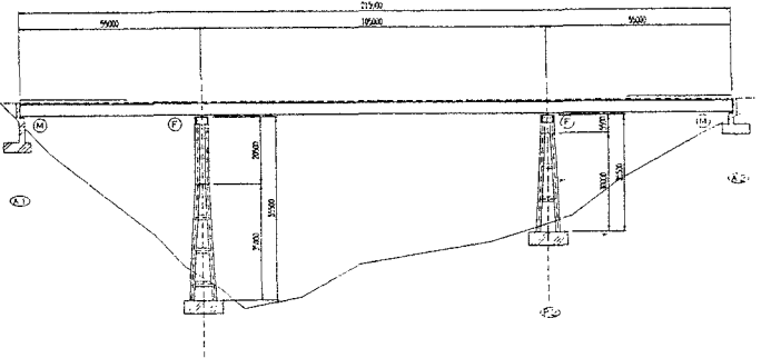
図-1 全体一般図
