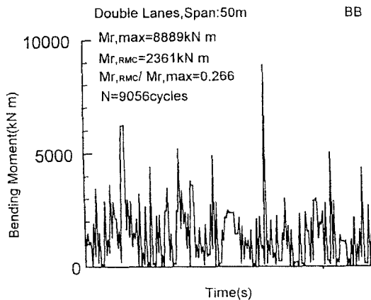
図-2 曲げモーメントの変動波形 (削除前)
