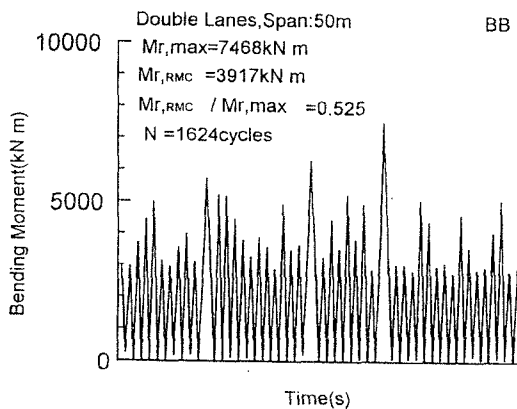
図-4 曲げモーメントの変動波形 (削除後)
