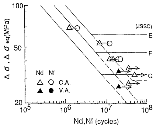
図-5 疲労試験結果
