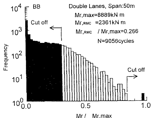
図-3 モーメント範囲の頻度分布 (削除前)
