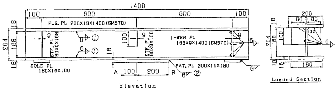
図-1 試験体の形状と寸法（寸法の単位はmm）
