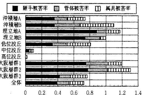
図1 地質分類別配水管被害
