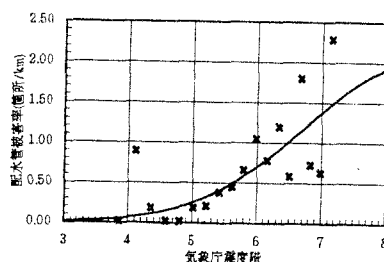
図4 気象庁震度階と配水管被害率
