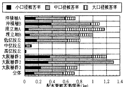
図2 口径別配水管被害
