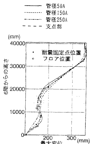
図-5 最大変位の比較 (SGP 内側)
