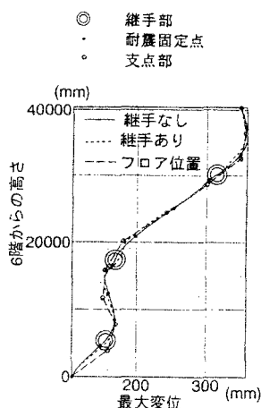
図-3 最大変位 (SGP 150A 内側)
