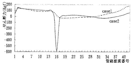
図5 最大ひずみ発生時刻のせん断力分布図
