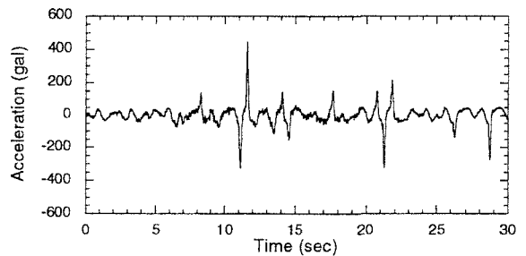
図4 桁の加速度応答波形
