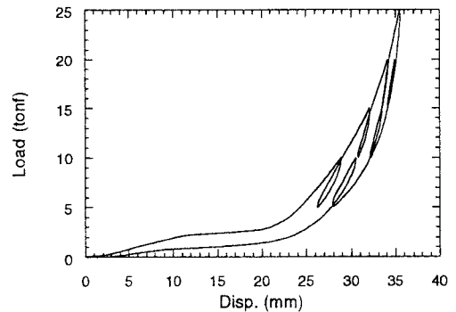
図 1 供試体の荷重－変位曲線
