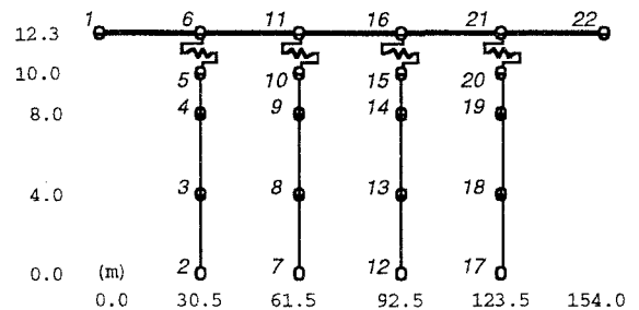
図3 5径間連続PC橋の有限要素モデル
