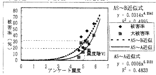
図-4 アンケート震度と橋脚被害の関係
