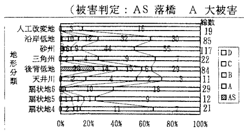
図-3 地形分類と橋脚被害の関係
