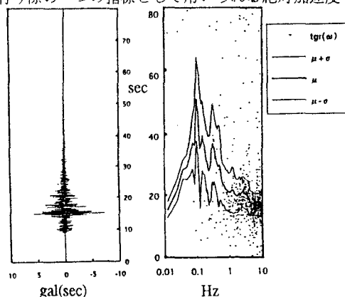
図1 鉾子で観測された地震の加速度時刻歴と群遅延時間
