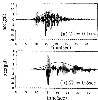
図2 鉾子で観測された地震の絶対加速度応答とその包絡線
