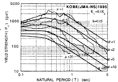
図6. 修正提案する保有耐力照査用震度
