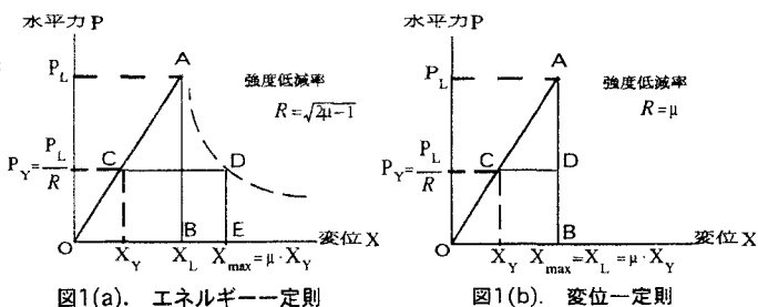
図1(a). エネルギー一定則
