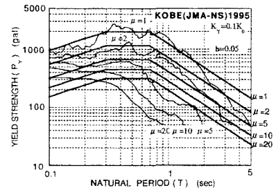
図5. 保有耐力照査用震度との比較
