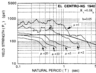
図3. エルセントロ記録の必要強度スペクトル
