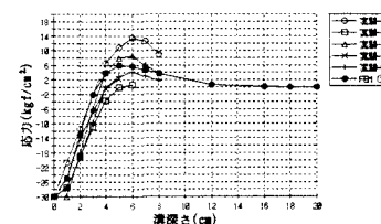
図-6 応力度-溝深さ関係
