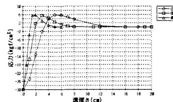
図-4 カッター径による比較
