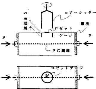
図-2 試験方法
