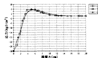
図-5 換算カッター径による比較
