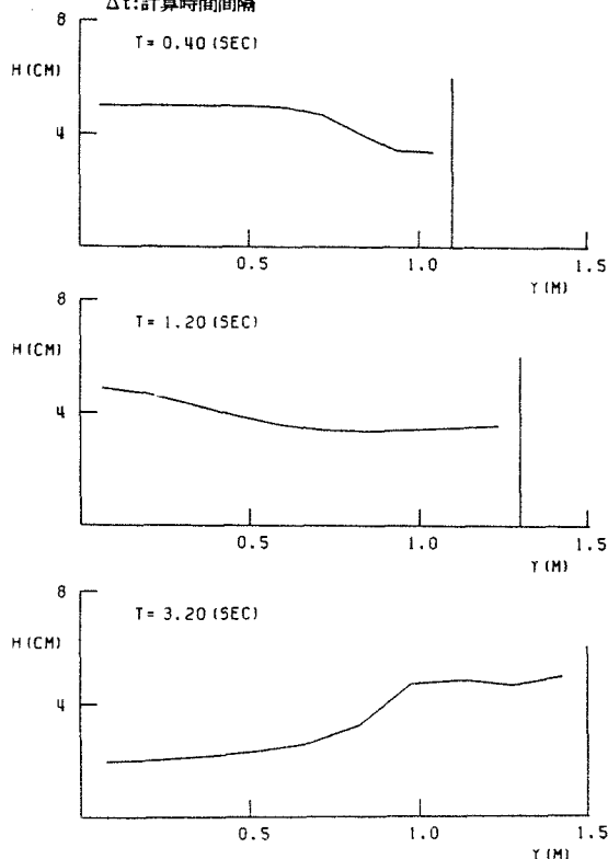
図-3 Run1-1の水面形
