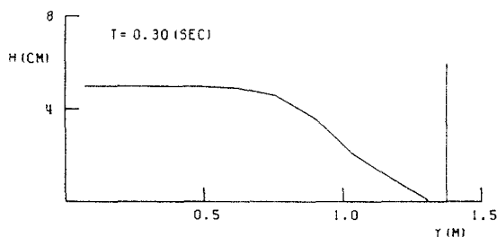
図-4 Run1-2の水面形
