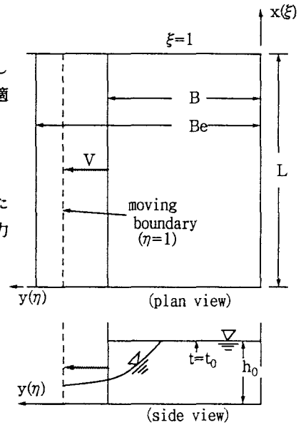
図-1 対象とする流れ
