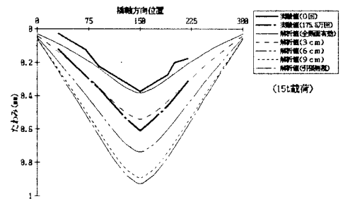
図-4 たわみ分布図(SB16)
