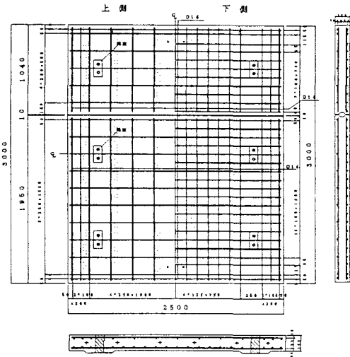
図-1 供試体(SB18)
