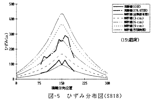
図-5 ひずみ分布図(SB18)
