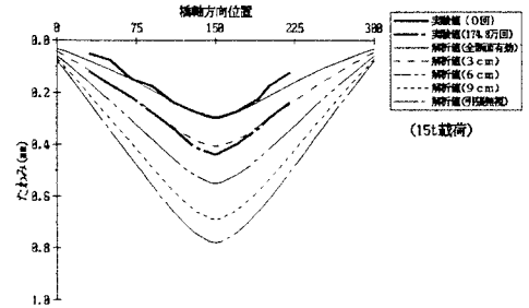
図-3 たわみ分布図(SB18)
