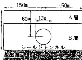
図3 解析モデル
