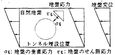
図2 地盤応力
