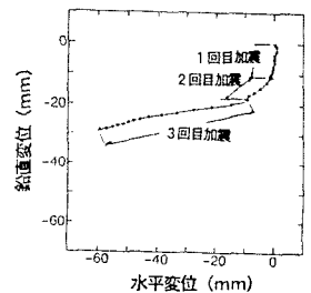
図4 測点1の位置の推移
