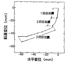
図5 測点3の位置の推移
