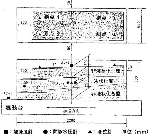
図1 モデルの構成と計測器の配置
