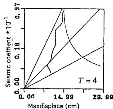
図4 降伏変位と最大変位の関係
