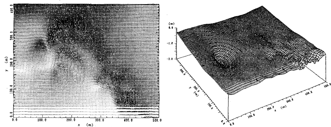
図4 (c) 流速ベクトルと水深の鳥瞰図（計算開始後198分）
