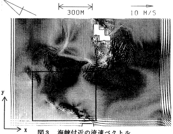
図3 海峡付近の流速ベクトル
