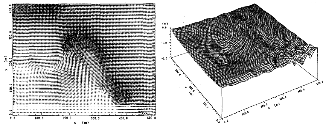
図4 (b) 流速ベクトルと水深の鳥瞰図（計算開始後197分30秒）
