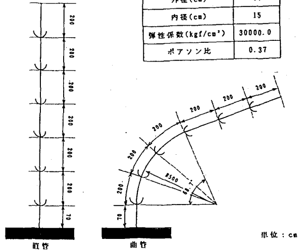
図5 解析モデル
