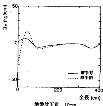
図3 円周方向せん断力
