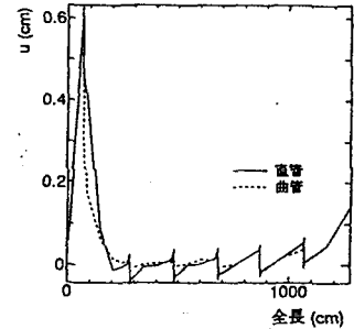
図6 管軸方向変位
