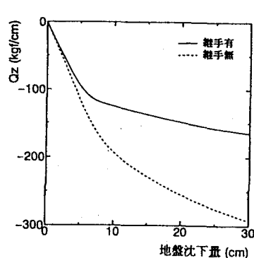
図4 半径方向せん断力
