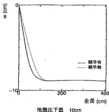
図2 鉛直方向変位
