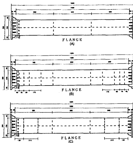
図1 供試体概略図
