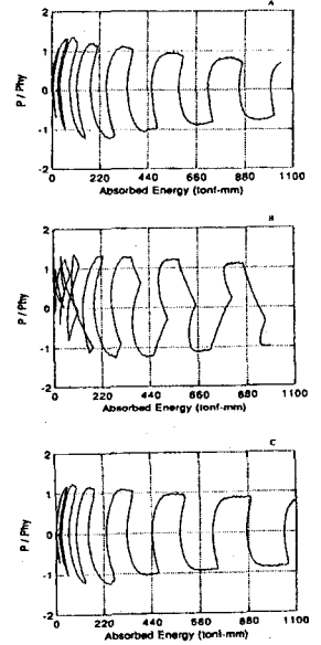
図4 耐荷力の劣化と履歴吸収エネルギー (静的繰返し載荷実験)
