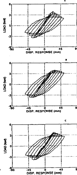
図3 変位-復元力関係 (静的繰返し載荷実験)
