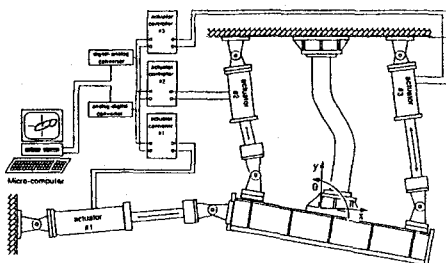
図2 載荷システム
