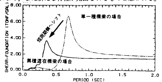
図-5 タイプ8橋梁群(橋脚番号6)の周波数応答関数と該当する部分の橋梁からなる単一種5径間橋梁の周波数応答関数の比較(基礎底面せん断力)
